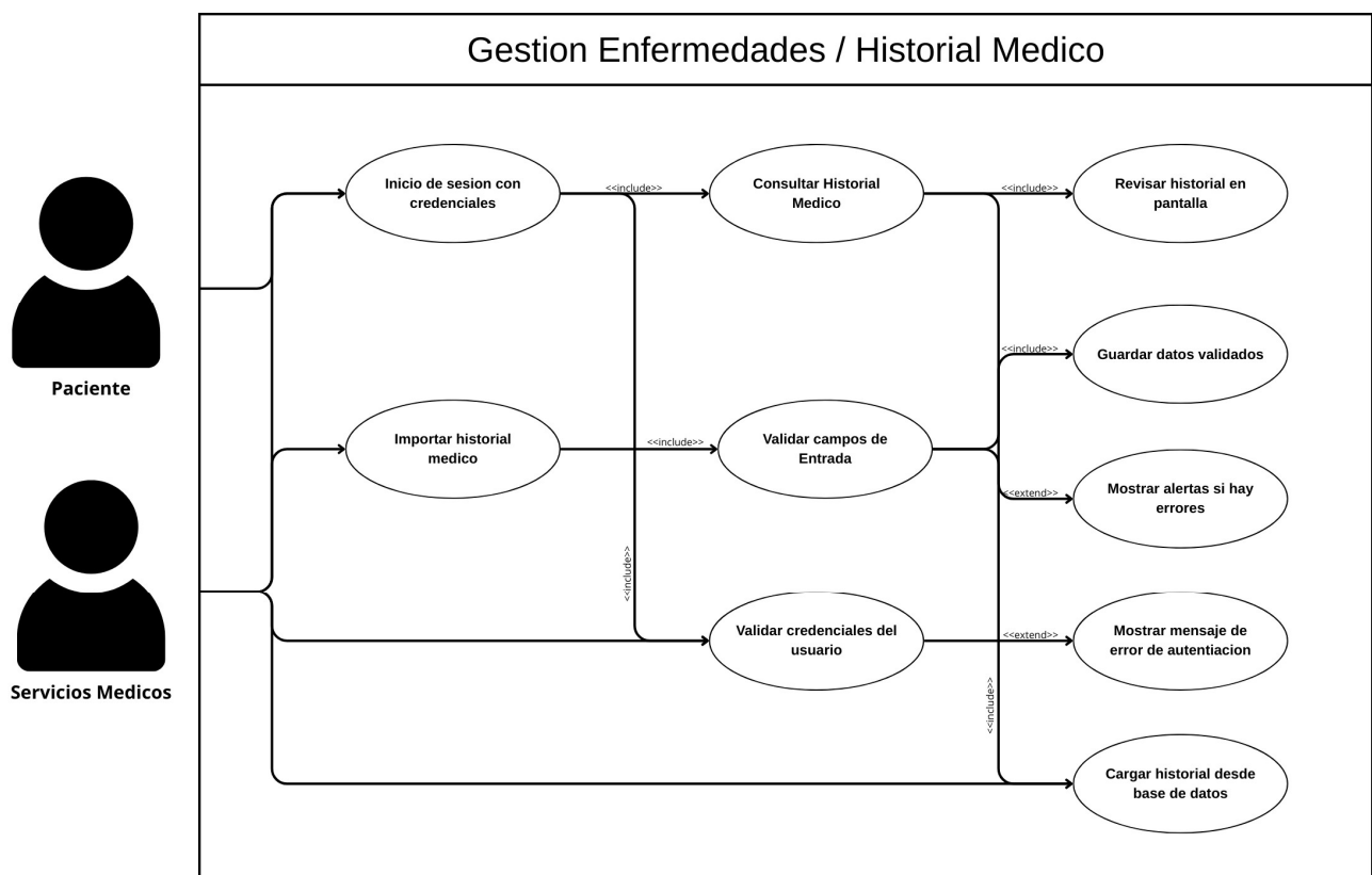
Diagrama de Caso de Uso (UML)
